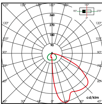
Silent asimétrica 1x28W
