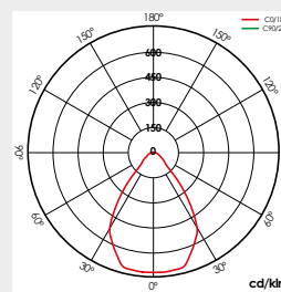
Superficie S069L0P Surface S069L0P Surface S069L0P Superficie S069L0P
