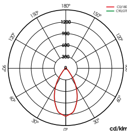
12W
