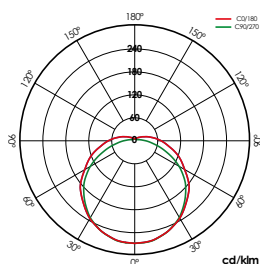
2x20W 1.200mm
