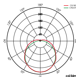
2x25W 1.500mm
